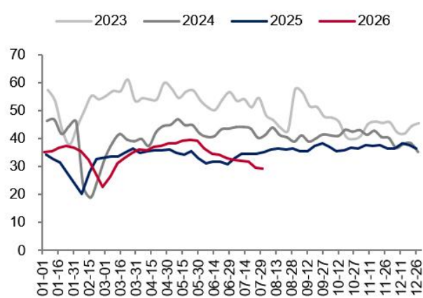
图表 36：样本洗煤厂（314 家）周平均产能利用率
