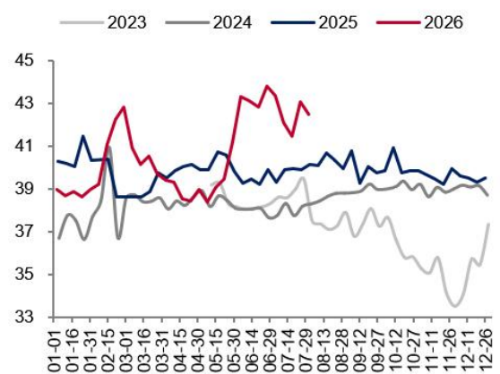
图表 40：523 家样本矿山精煤洗出率
