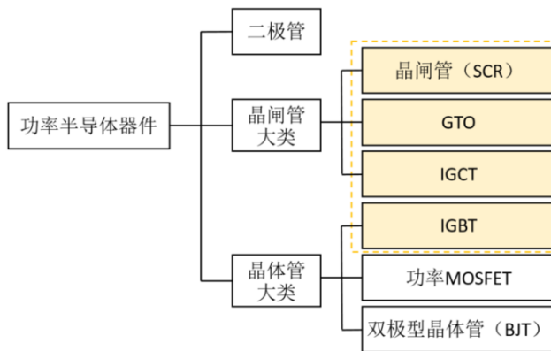
图1：功率半导体器件主要分为二极管、晶闸管、晶体管三类
