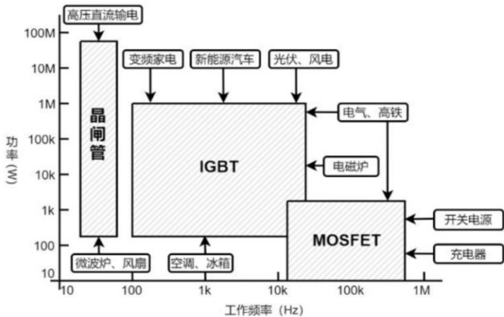
图2：各类型功率半导体器件应用场景
