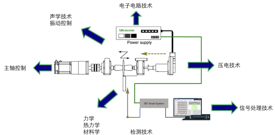
图表34：超声波滚动焊接技术原理图
