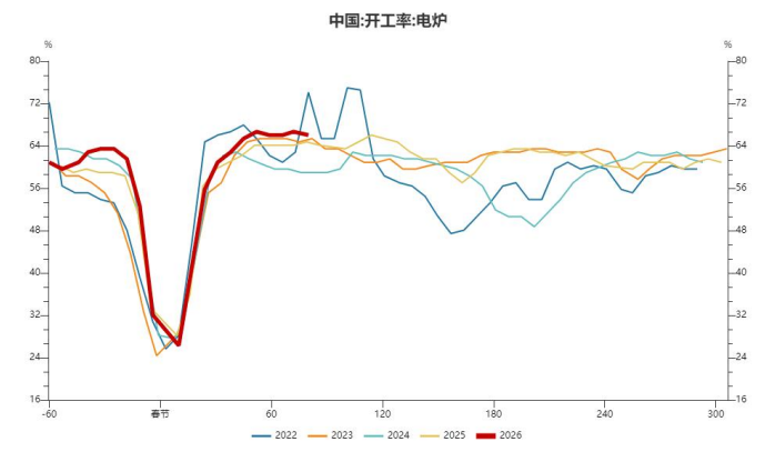
图 11：电炉开工率下降
