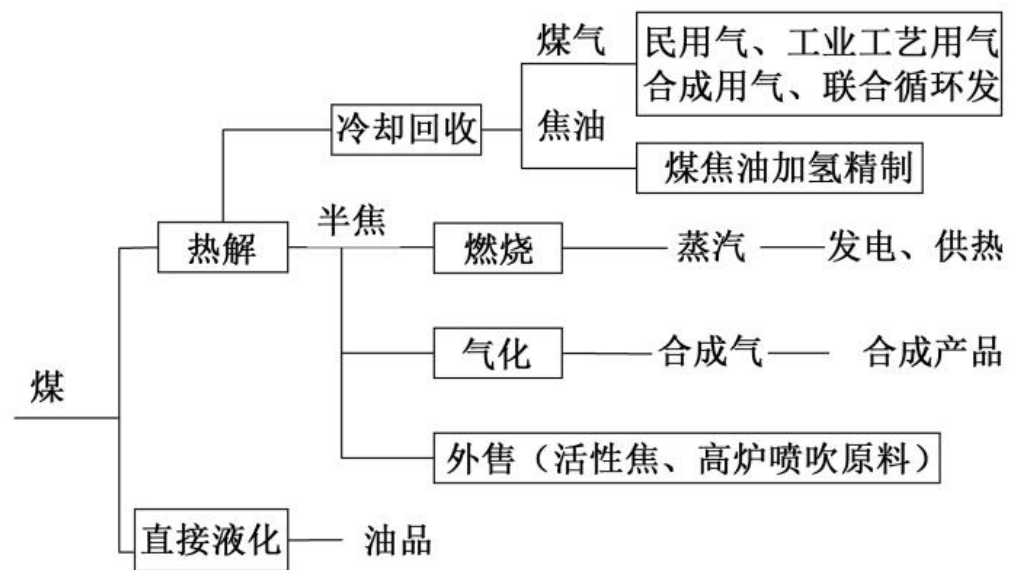
图表 30：煤分质利用技术路线图
