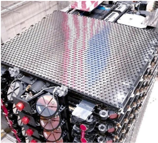
图9：SpaceX 星链 V2 mini 卫星
