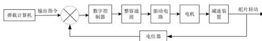
图22: 弹载舵机系统工作原理图
