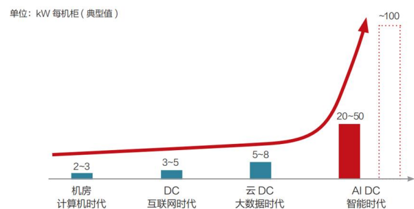
图39: 不同时代数据中心机柜典型功率
