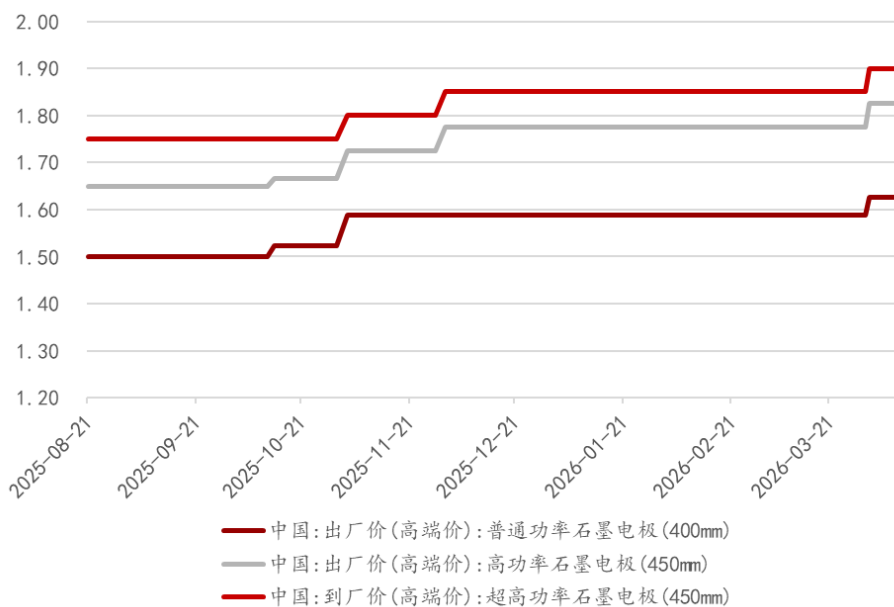
图表11: 石墨电极价格变化趋势（万元/吨）
