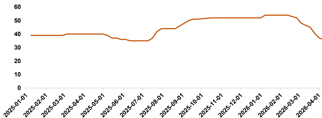
图 19: 多晶硅 (致密料) 周均价 (元/千克)
