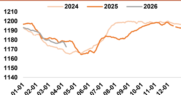
图 17: 二滩水库水位 (米)
