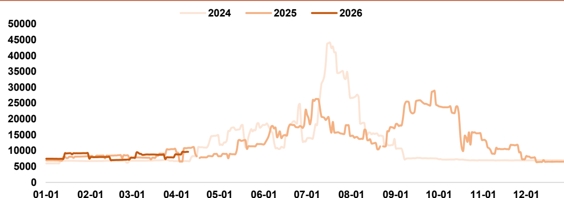
图 14: 三峡水库出库流量 (m³/秒)
